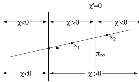
Fig. 21.5. The parameter \chi .
